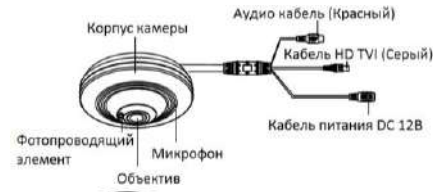
Рисунок 1-26 Панорамная камера
